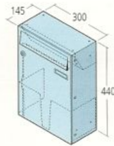
Mail box 300 x 440 x 145 mm
