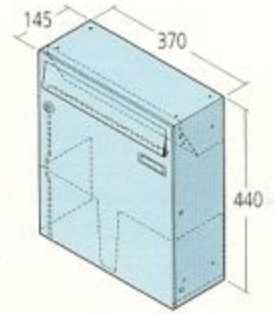
Mail box 370 x 440 x 145 mm
